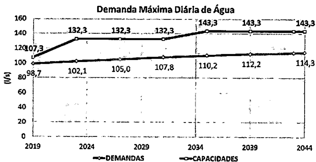
Figura 1 – Evolução da Demanda Máxima Diária de Água
