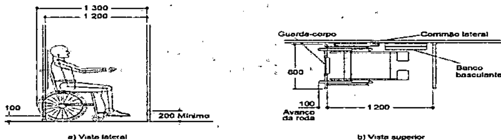
Figura 2 — Referências dimensionais da área reservada
